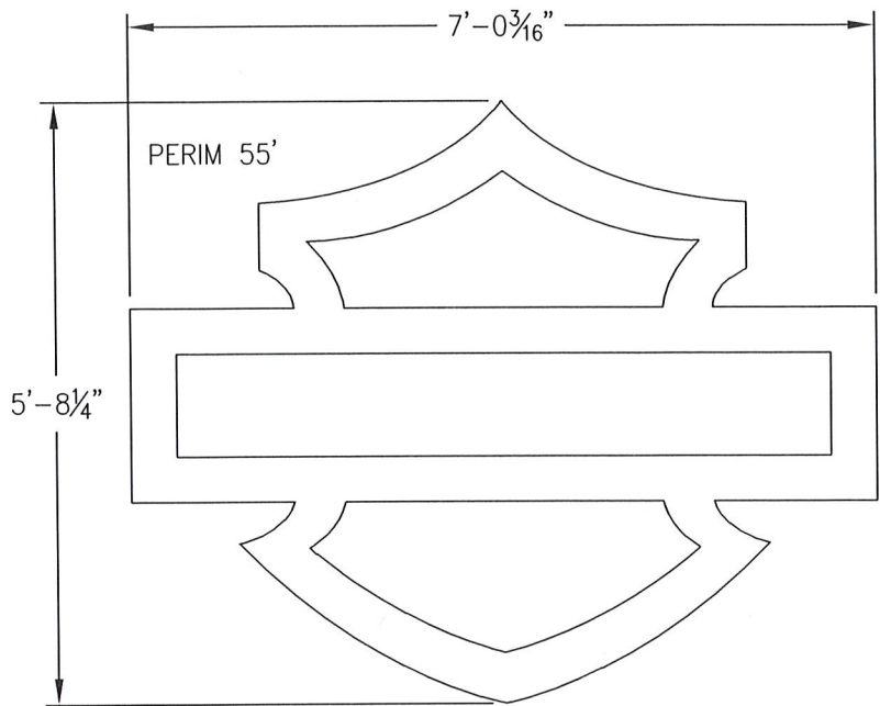
ELEVATION SCALE: 1/2"=1'-0"
