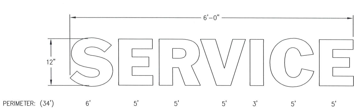
ELEVATION
