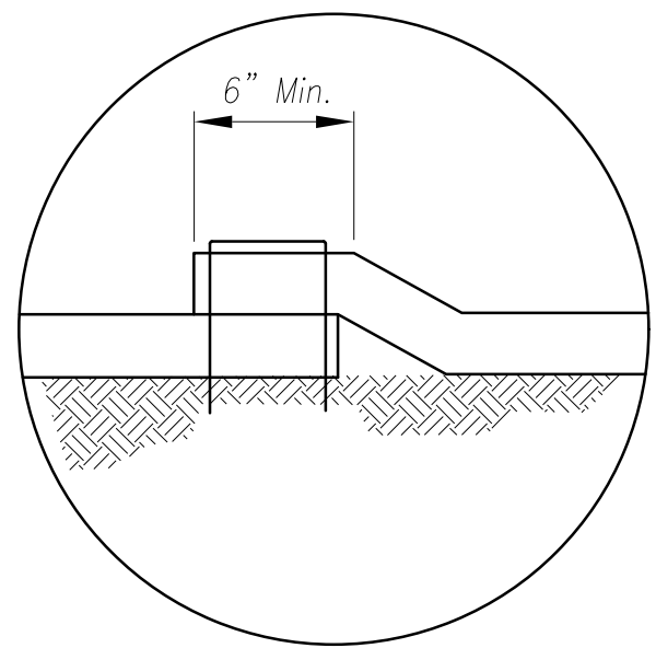
Longitudinal Seam
