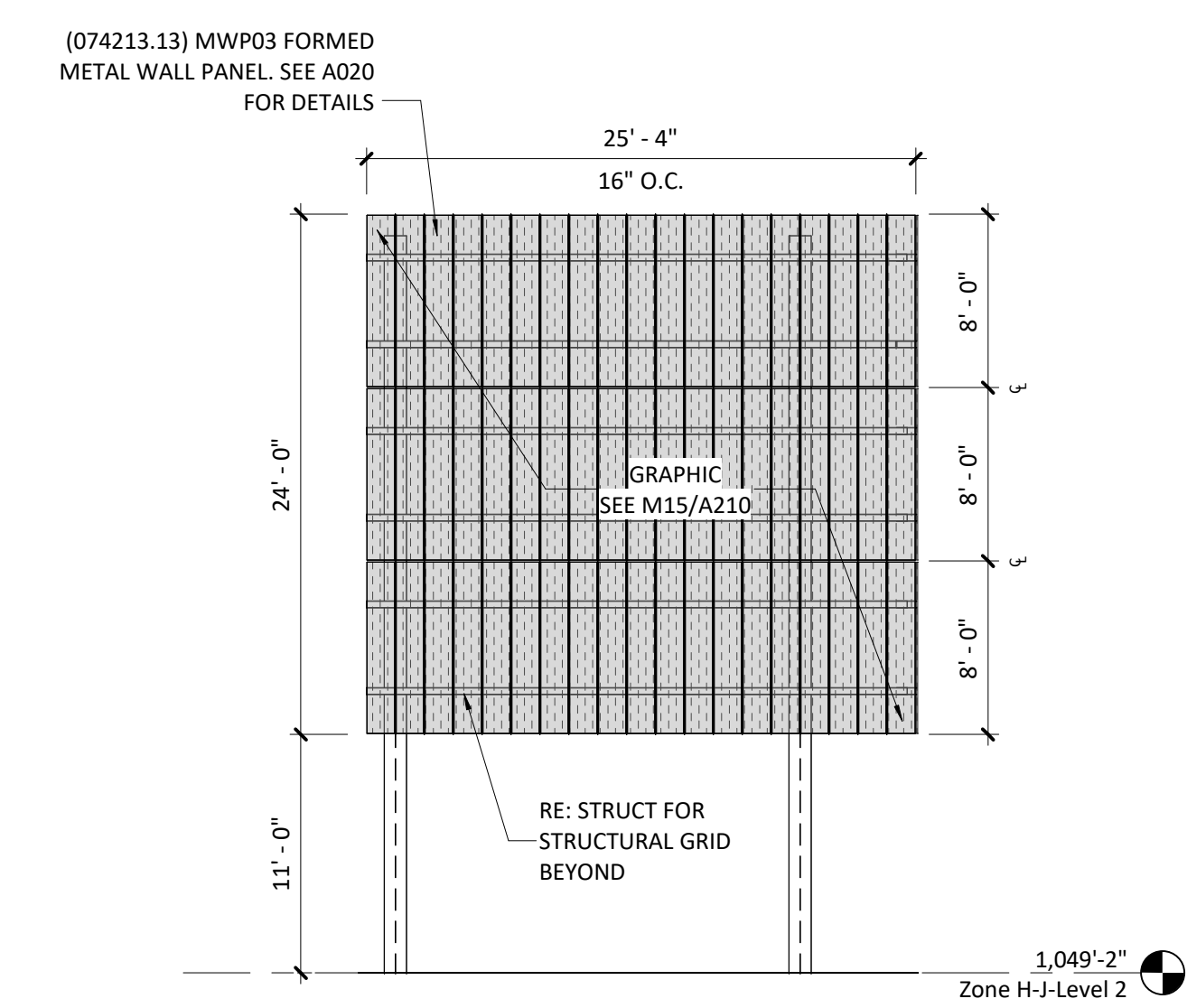
Scrim West 1/8" = 1'-0"
