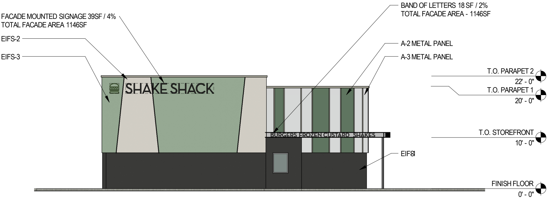
1 EXTERIOR ELEVATION - WEST - BOL N.T.S.
