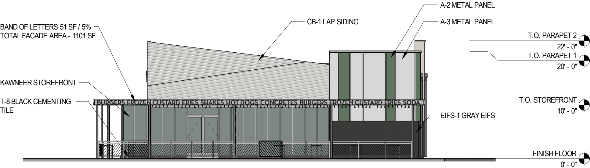
1 EXTERIOR ELEVATION - EAST - BOL N.T.S.
