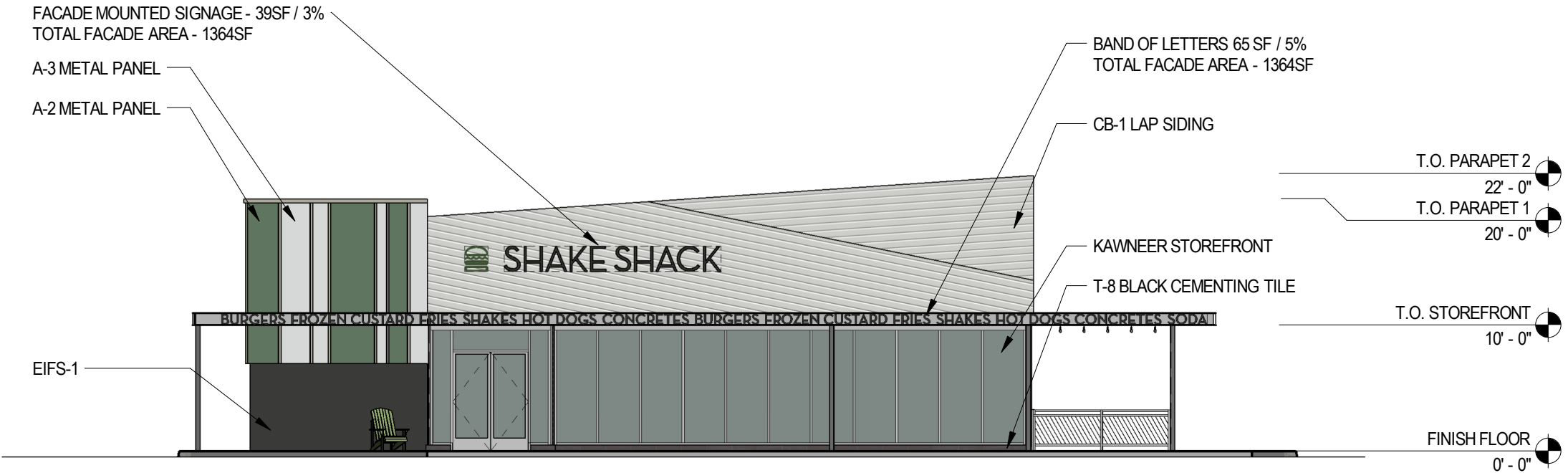
2 EXTERIOR ELEVATION - SOUTH - BOL N.T.S.
