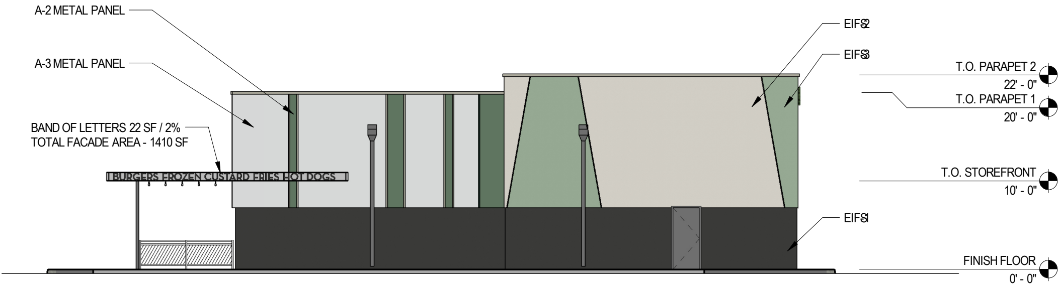
2 EXTERIOR ELEVATION - NORTH - BOL N.T.S.
