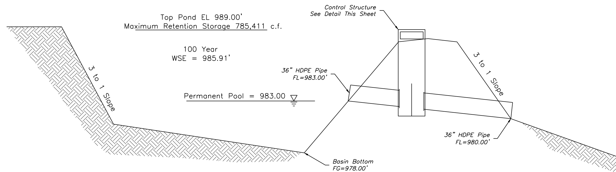
SECTION VIEW N.T.S.
