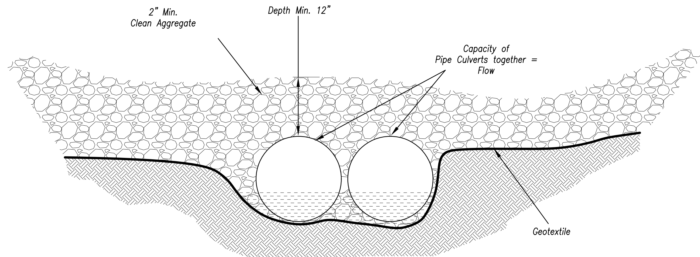
ELEVATION
