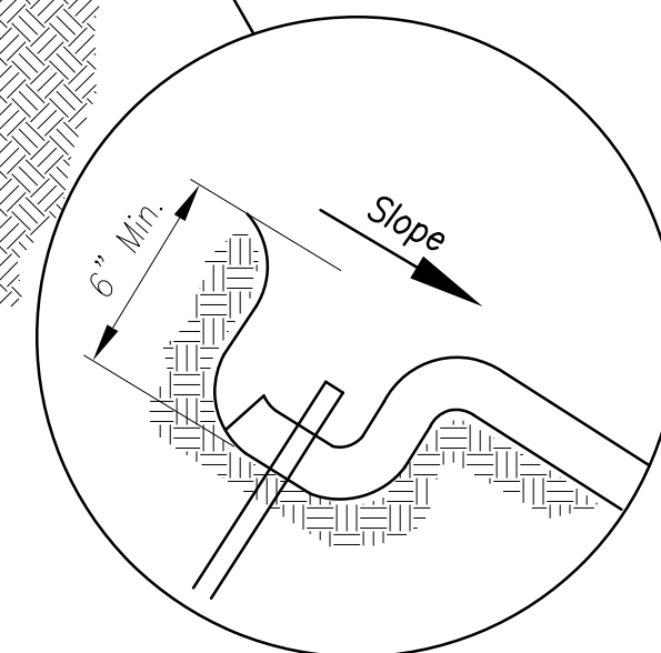
Edge Anchor
