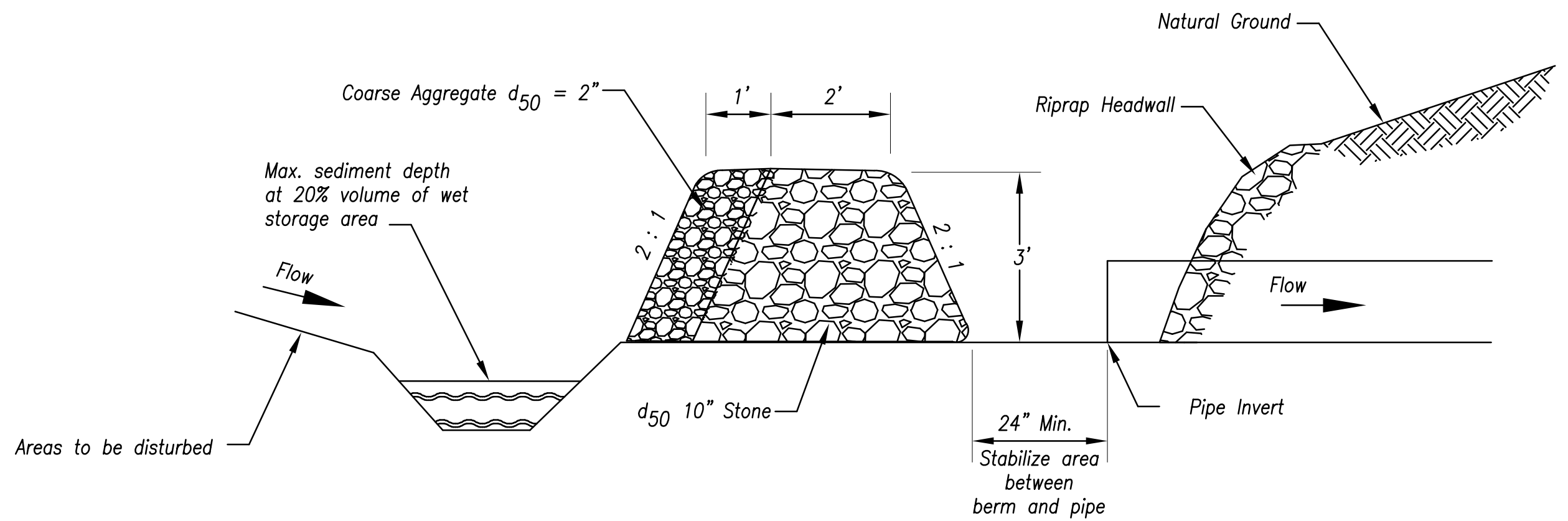
Section A-A
