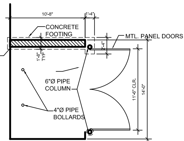
3 TRASH ENCLOSURE SCALE: 1/100" = 1'-0"
