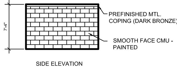
3 TRASH ENCLOSURE SCALE: 1/100" = 1'-0"
