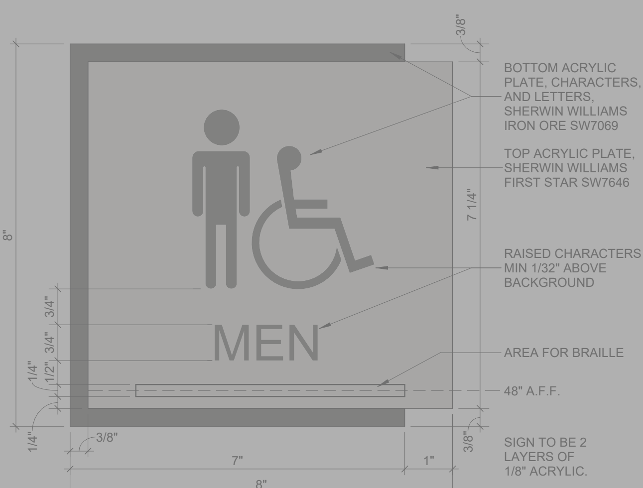
E7 SIGNAGE - TOILET MEN (M-RR) 6" = 1'-0"
