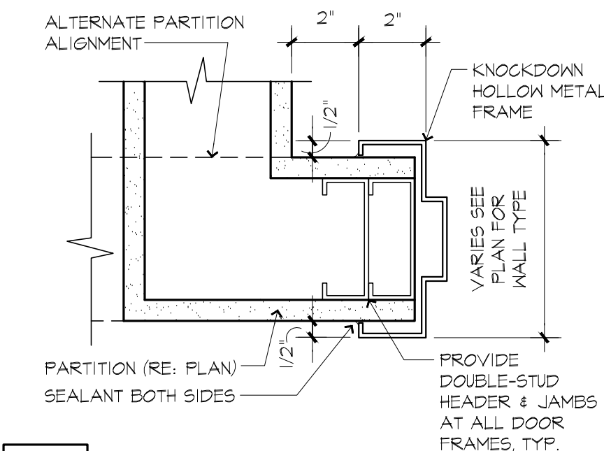
P2 DOOR DETAIL
