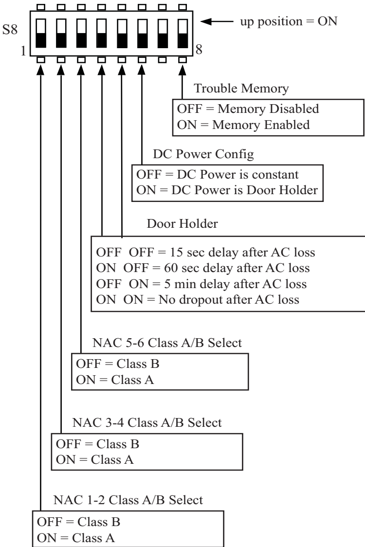
DWG# 3590-16
