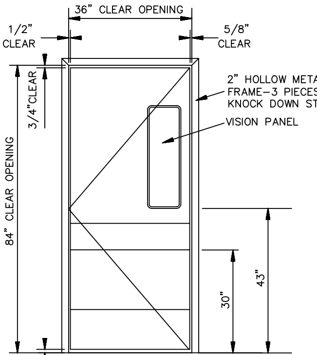
TYP. 3'x7' HM SWING DOOR & FRAME
