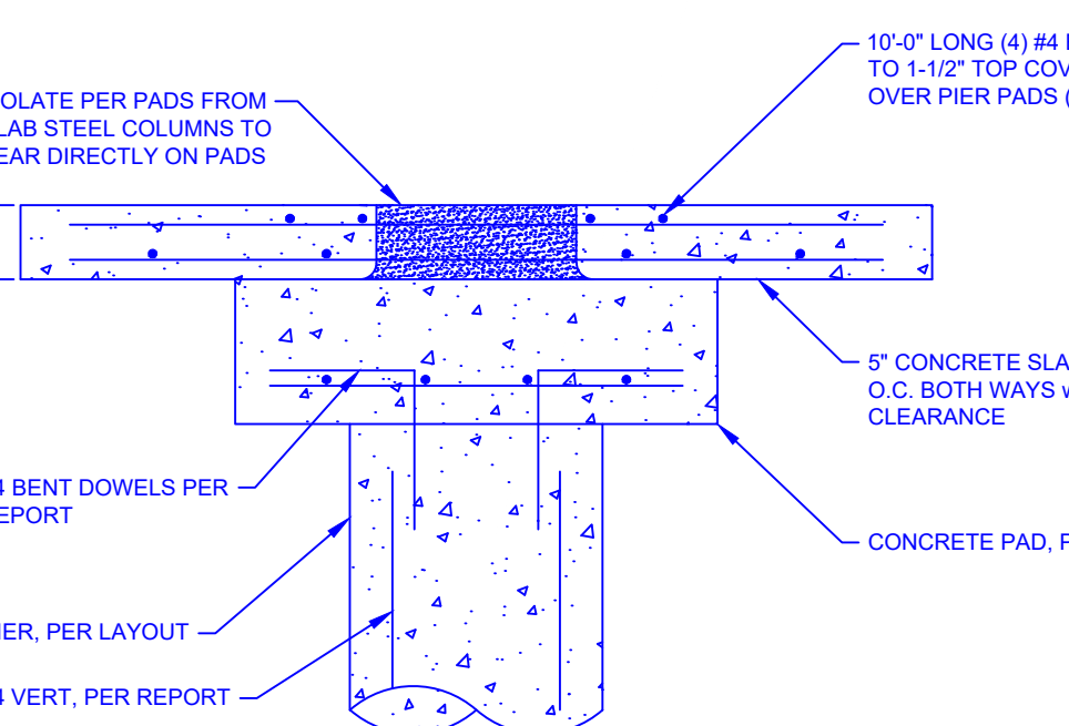
4 S2.1 PIER / PAD DETAIL N.T.S.
