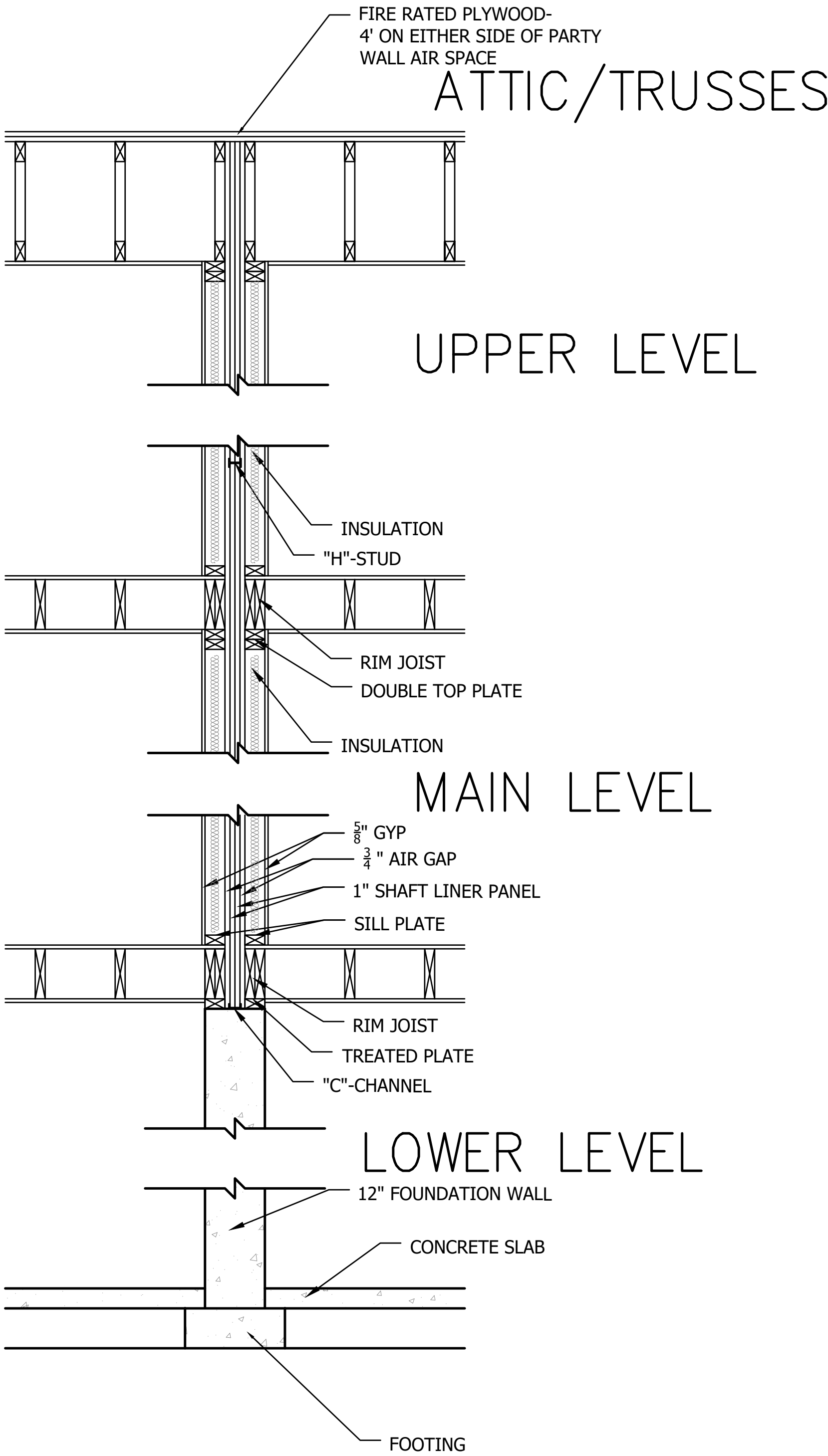
PARTY WALL DETAIL 2 SCALE: N.T.S.
