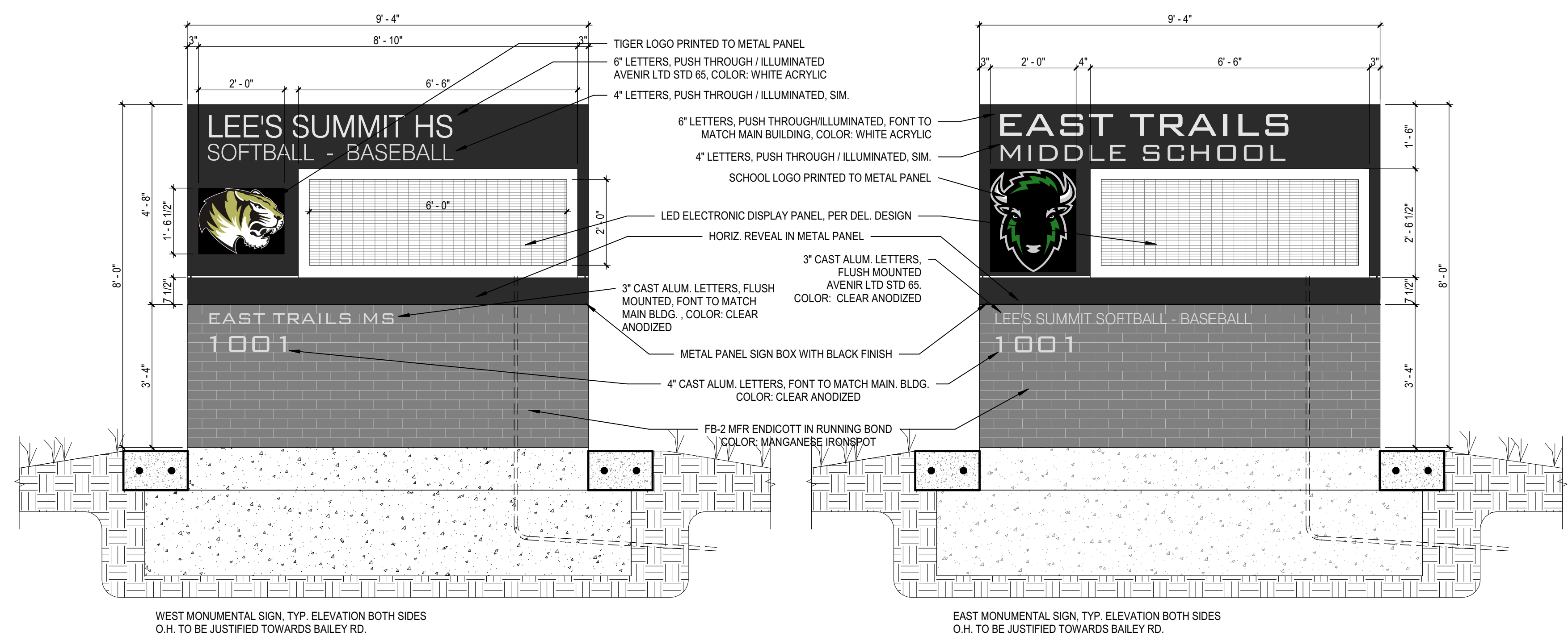
1 MONUMENT SIGN SCALE: 1/2" = 1'-0"
