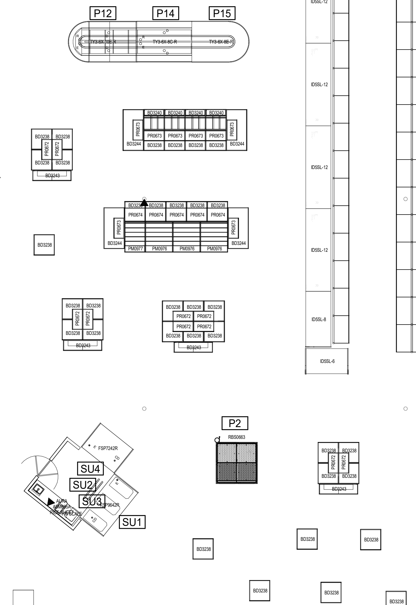
3 PRODUCE SCALE: 1/8" = 1'-0"
