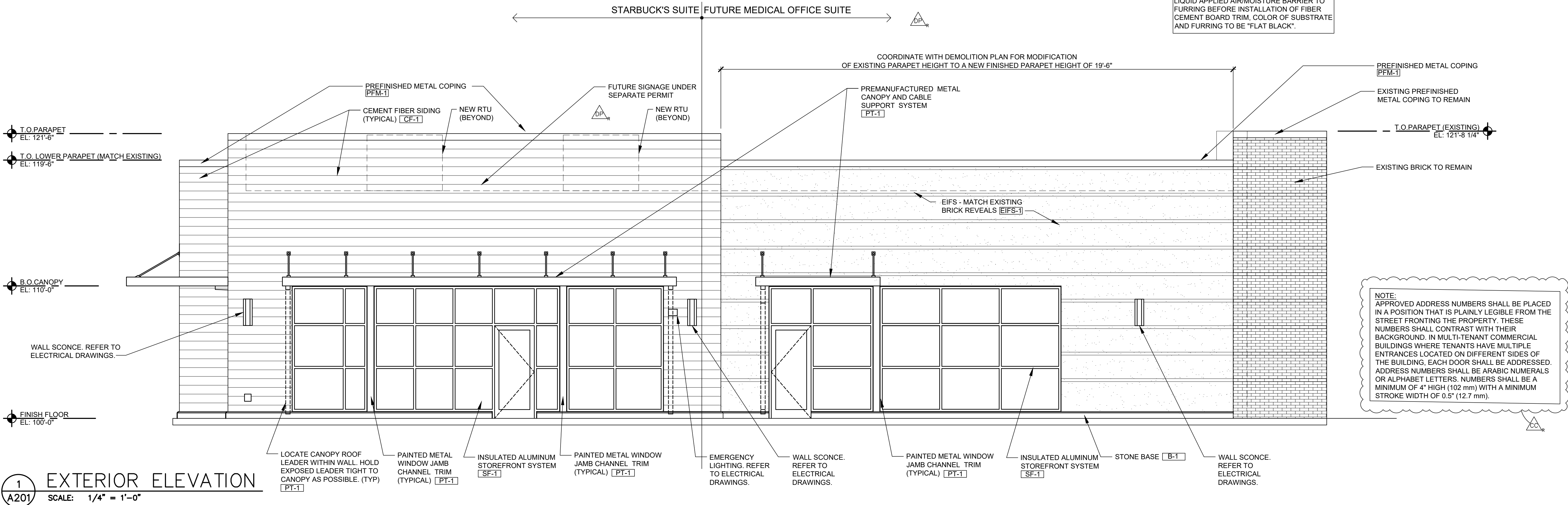
2 EXTERIOR ELEVATION A201 SCALE: 1/4" = 1'-0"
