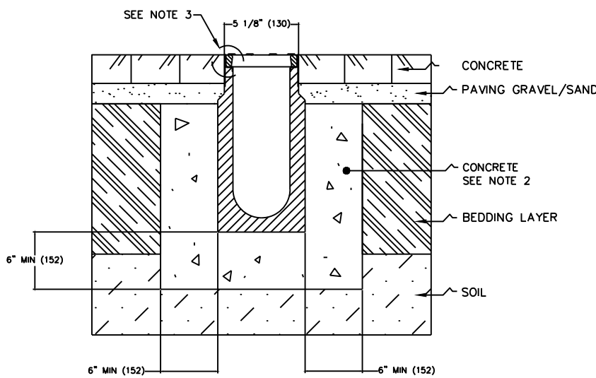
TRENCH DRAIN DETAIL N.T.S.
