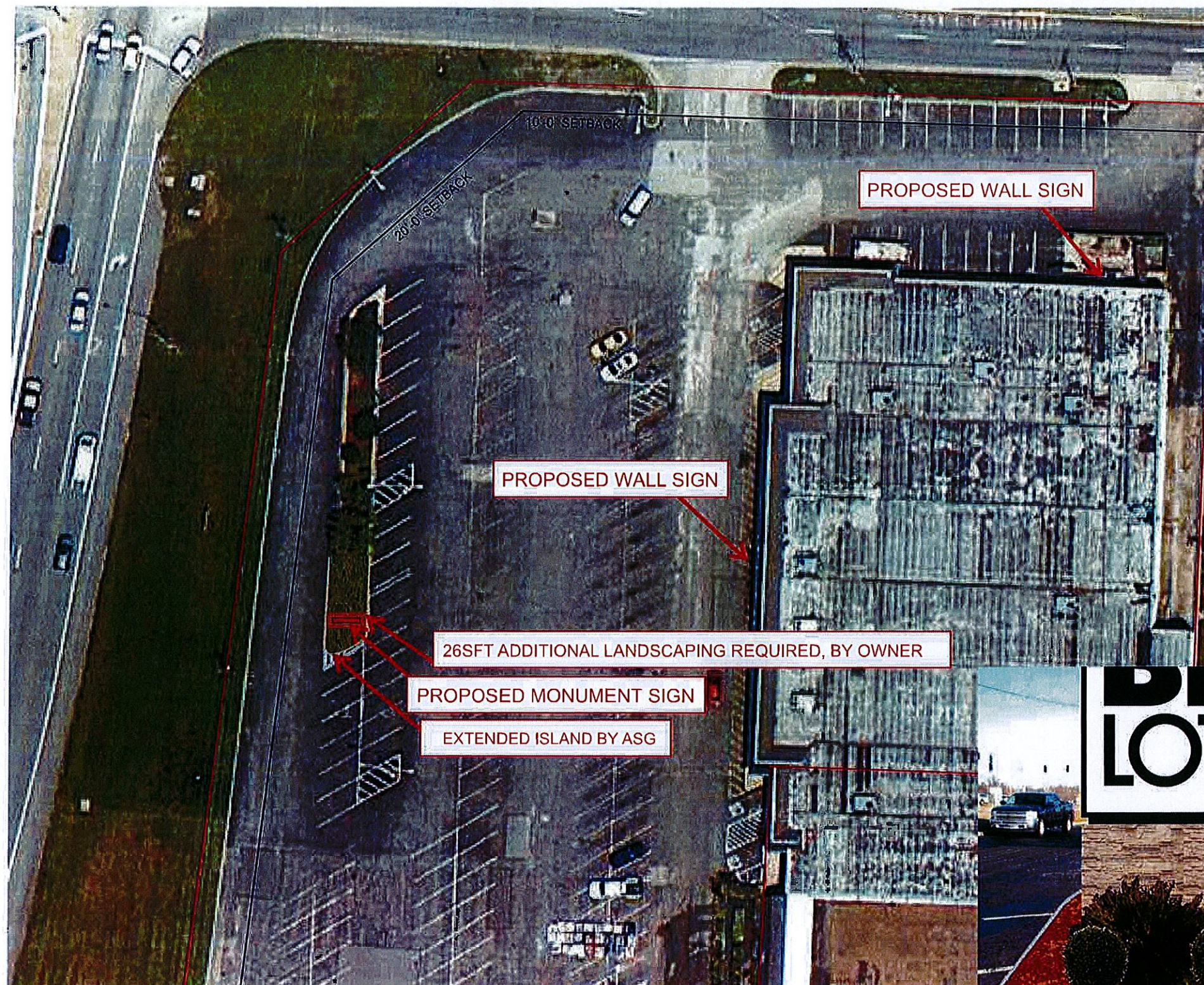
SITE MAP- OPTION A SCALE: NTS
