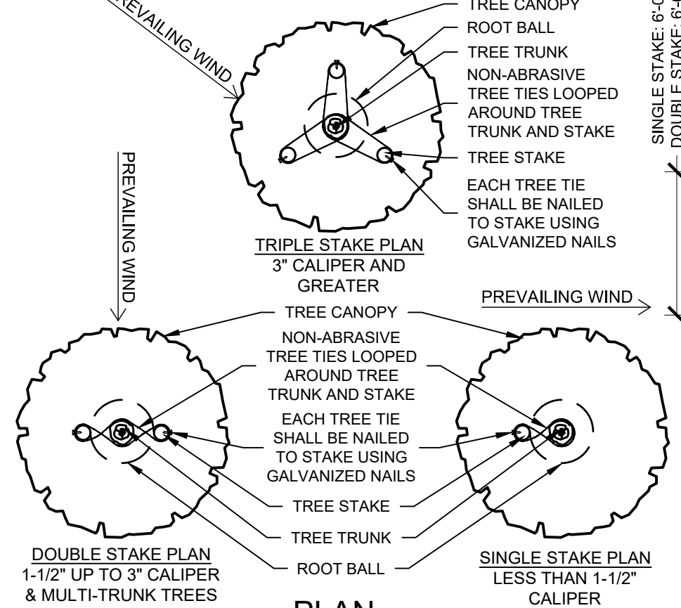
2 TREE STAKING N.T.S.
