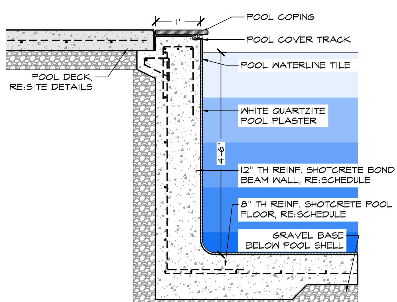
6 DEEP END SCALE: 3/4" = 1'-0" SECTION
